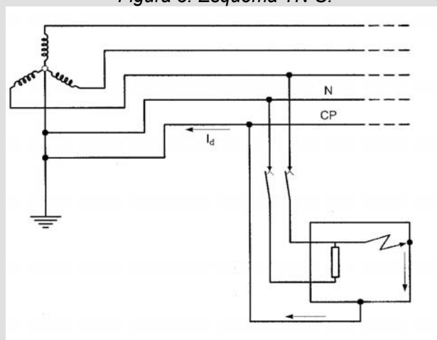
Figura 3. Esquema TN-S.
