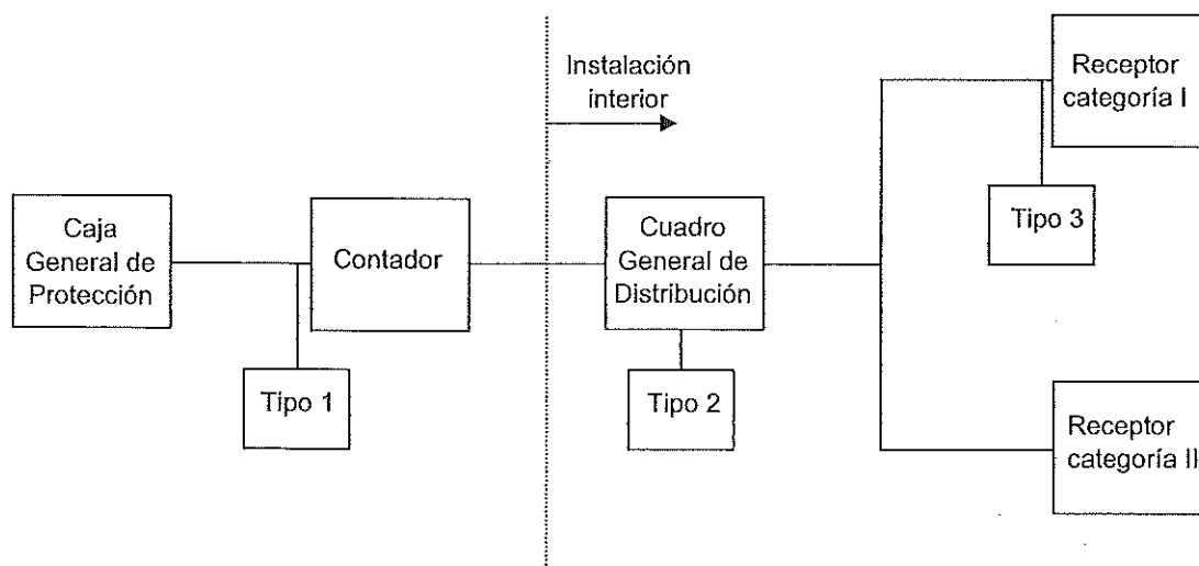
Ejemplo de instalación que incluye los tres tipos de dispositivos de protección contra sobretensiones transitorias.
